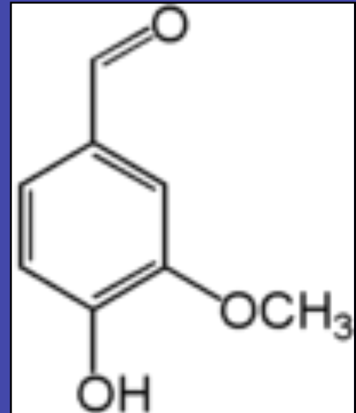
Vanilya C 8 H 8 O 3
